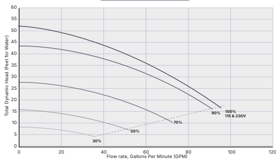
inverFLOW M200
