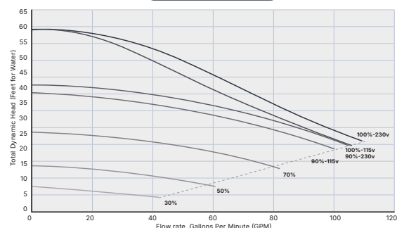
inverFLOW M150
