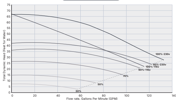
inverFLOW M200
