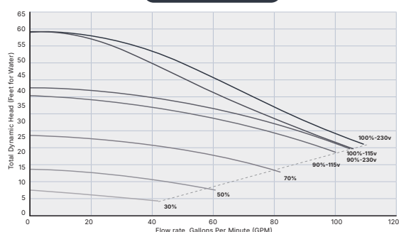
inverFLOW M150
